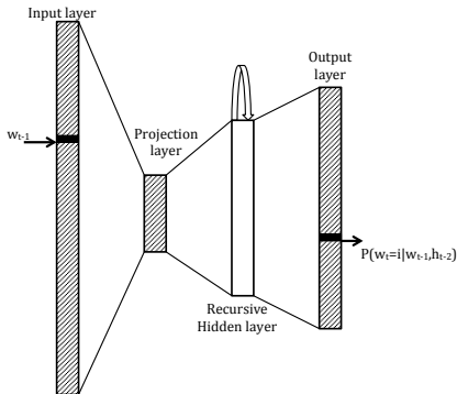
Yinelemeli sinir ağı
