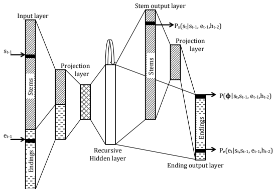
Sondan eklemeli diller için önerilen yinelemeli sinir ağı 23
